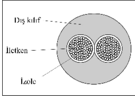
Şekil 5.2: H05VV-F kablo kesiti
