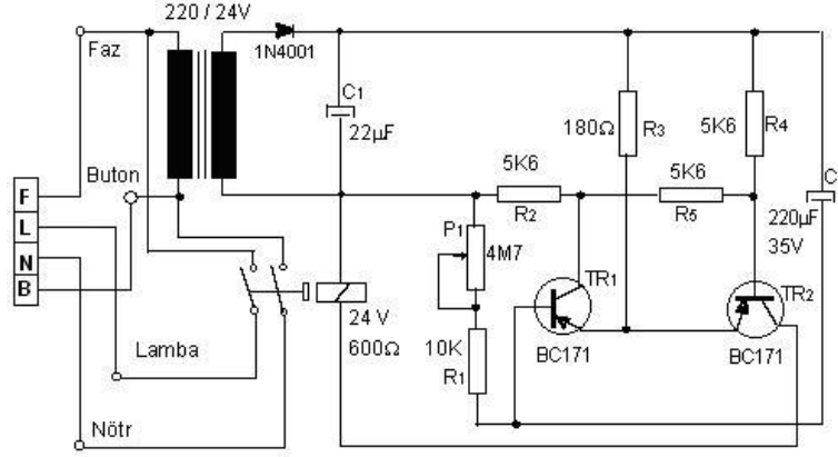
Şekil 2.1: Elektronik merdiven otomatiği devre bağlantı şeması
