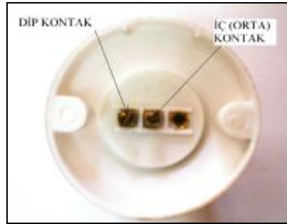
Resim1.40: Dyuun bağlantı vidaları
