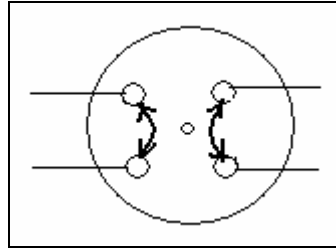
Şekil 1.9 : Ara vaviyen anahtar iç yapı bağlantı şekli
