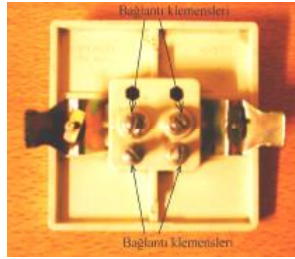
Resim 1.34: Ara vaviyen anahtarın arkadan görünüşü
