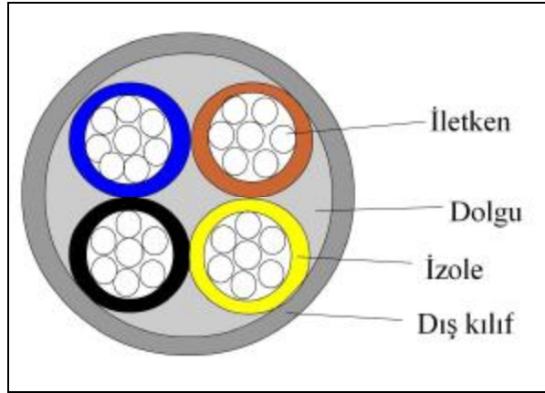
Şekil 5.1: NVV kablo kesiti
