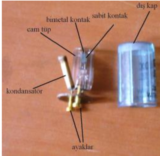
Resim 4.8: Starterin iç yapısı
