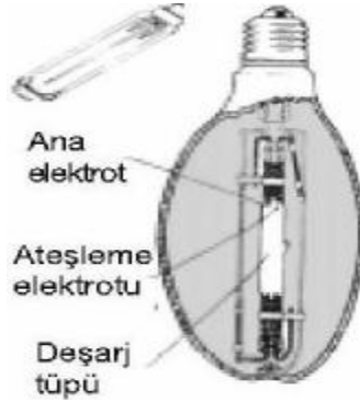
Şekil 1.3: Civa buharlı ampul
