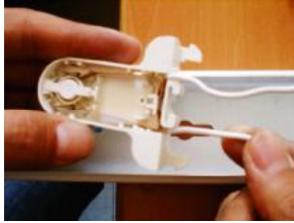
Resim 4.22: Soketin diğere ucunun bağlantısı
