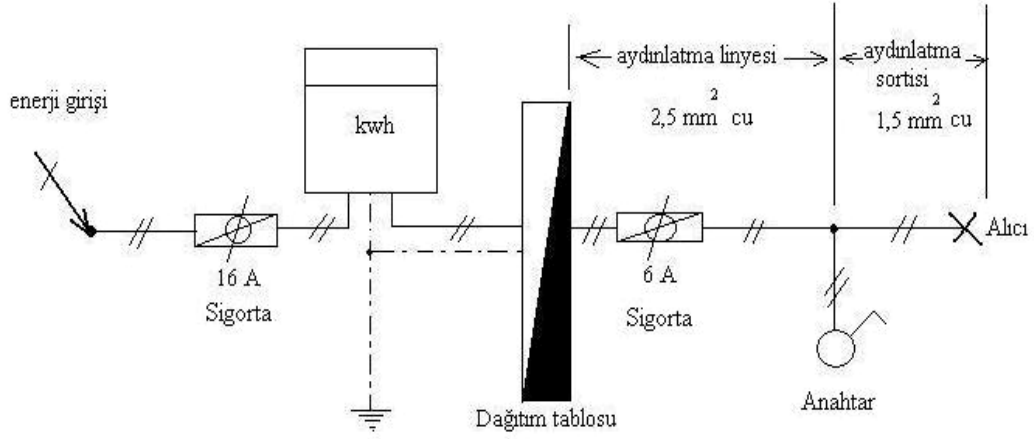
Şekil 1.1: Aydınlatma linyesi ve aydınlatma sortisi
