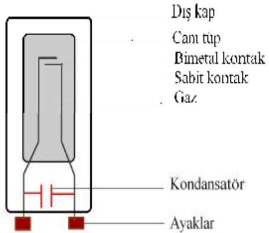
Şekil 4.7: Starterin iç yapı şekli
