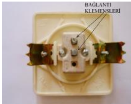
Resim 1.23: Sıva altı anahtarın arkadan görünüşü
