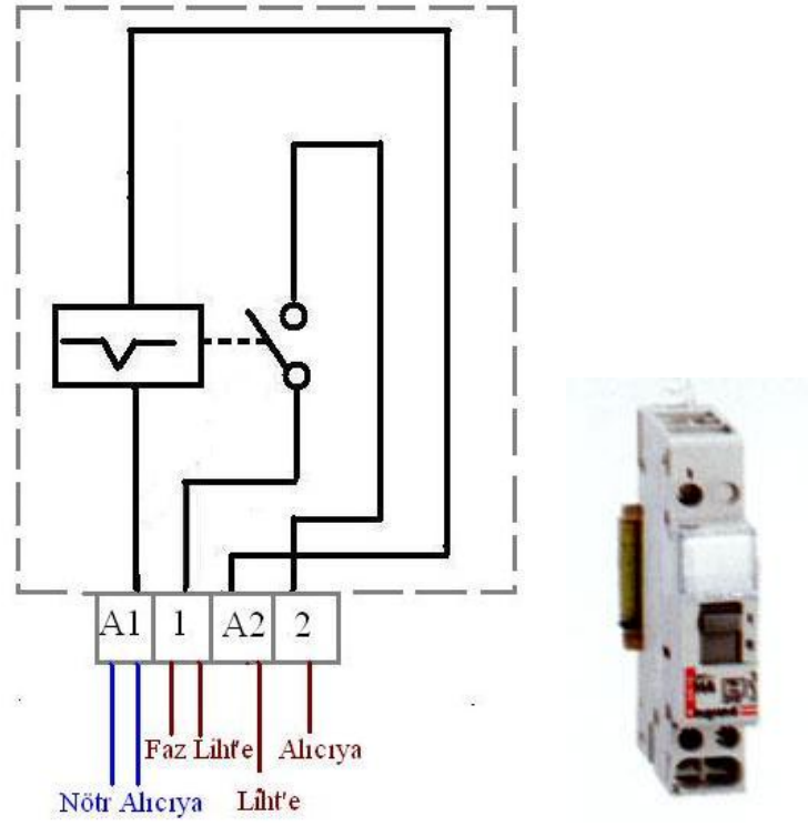
Şekil 1.10: İmpuls röle (darbe akımlı) klemens bağlantısı
