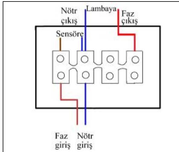
Şekil 2.3: Hareket sensörünün klemens bağlantısı
