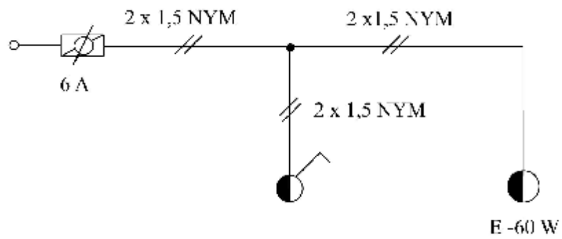
Şekil 5.7: Nemli yer malzemesi ile adi anahtar tesisatı kapalı şema
